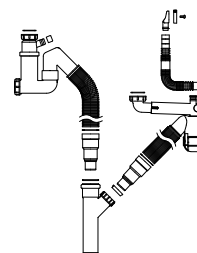
Dubbelt vattenlås med gängad anslutning
