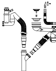
Dubbelt vattenlås med gängad anslutning och korgventil
